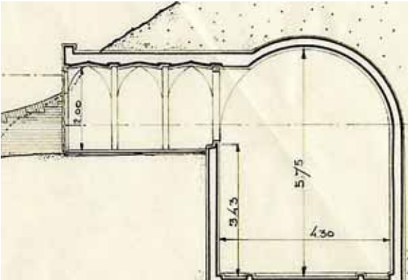
De opmetingstekening van de ijskelder uit 1950.
